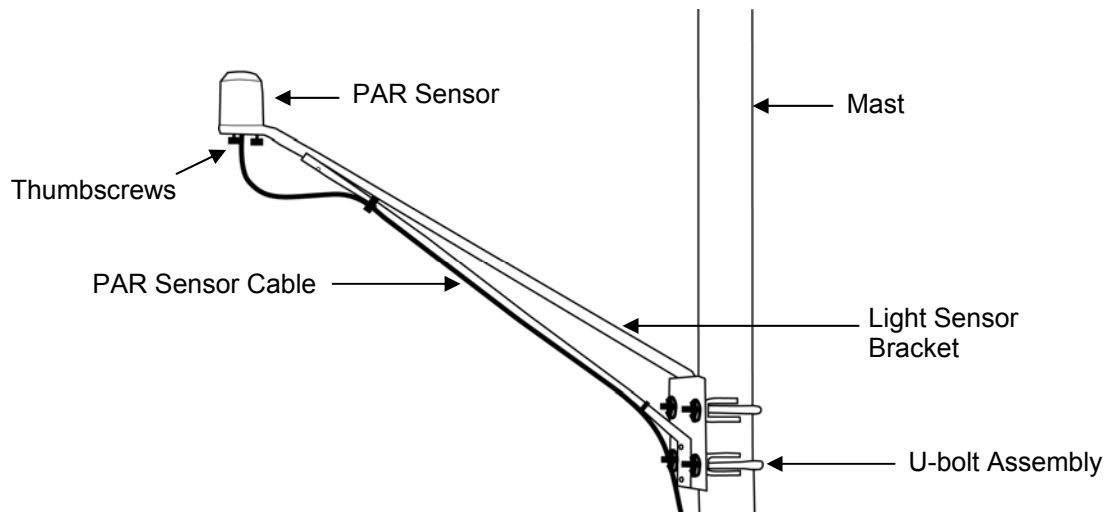
Figure 2: PAR Smart Sensor Bracket Mounting
